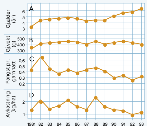
Figur 2. Samanstilling av ulike resultat frå undersøkingane i Aursjoen frå 1981 til 1993: gjennomsnittleg alder på 40 mm garn (A), gjennomsnittleg vekt (B), fangst pr. garnnett i kg (C), avkastning i kg pr. hektar (D)
